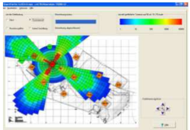
Evaluation des zones d'effets prenant en compte la structure du magasin de stockage
